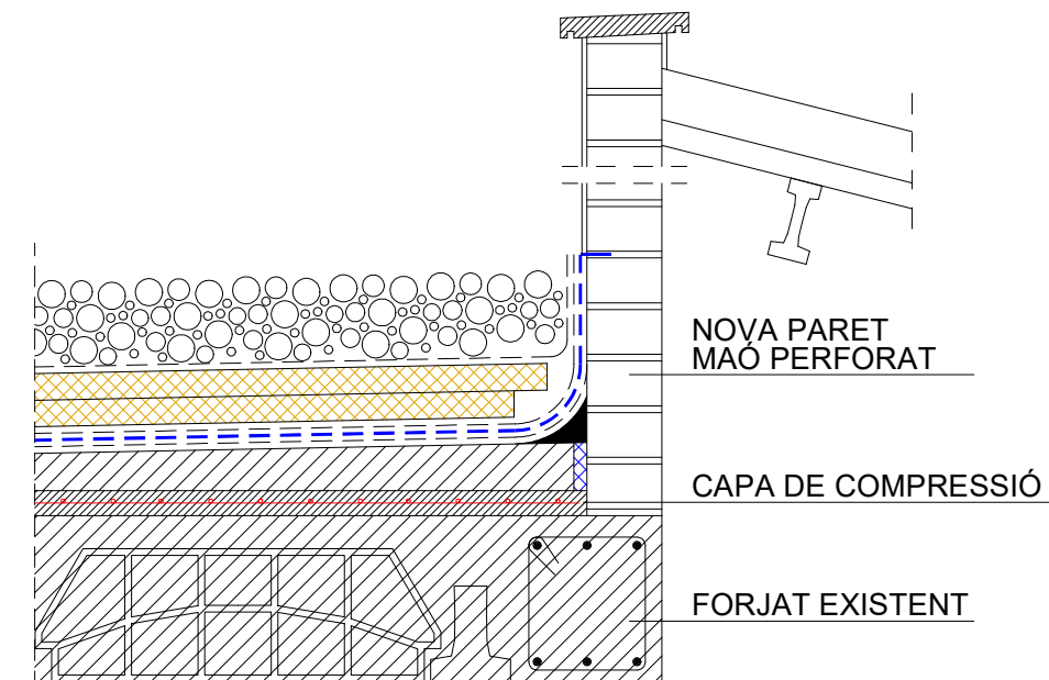
DETALL CONSTRUCTIU E: 1/20
